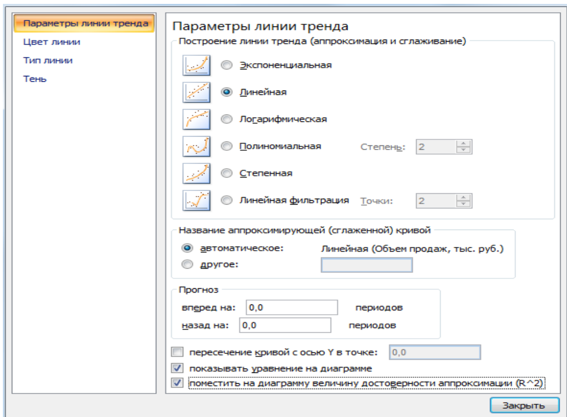
Рис. 2. Оконная форма меню задания параметров линии тренда
