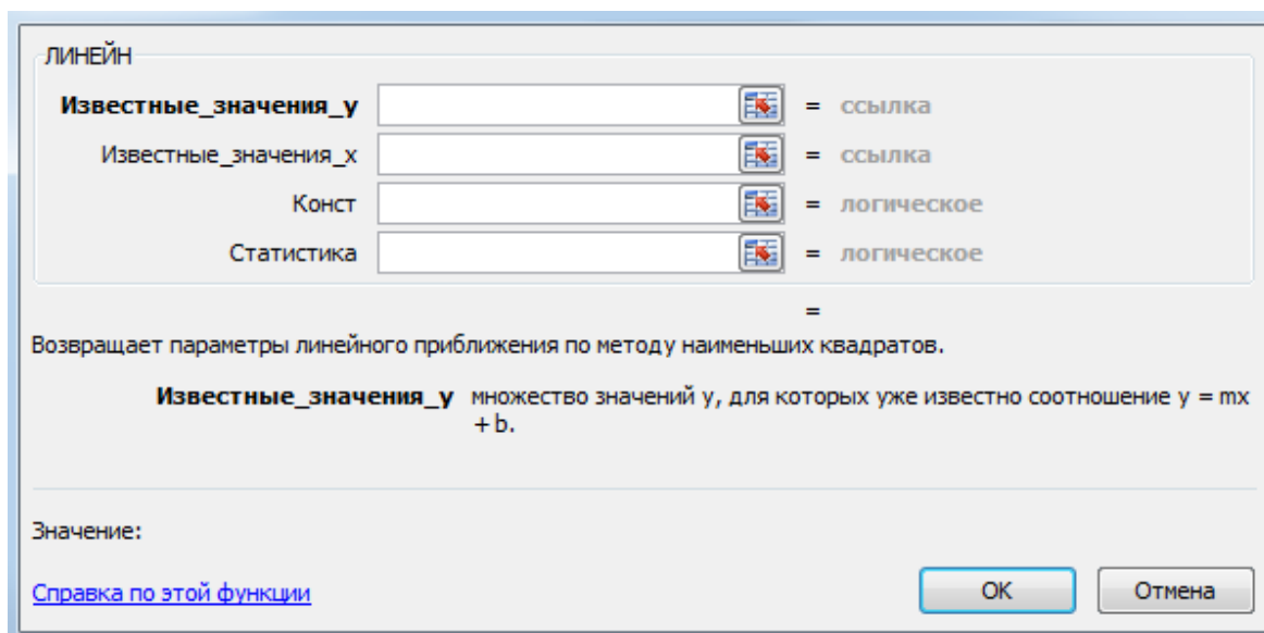
Рис. 5. Оконная форма встроенной функции Microsoft Excel «ЛИНЕЙН», возвращающей параметры уравнения линейной множественной регрессии
