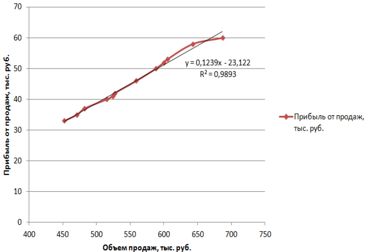
Рис. 4. График функциональной зависимости прибыли от продаж, от объема продаж
